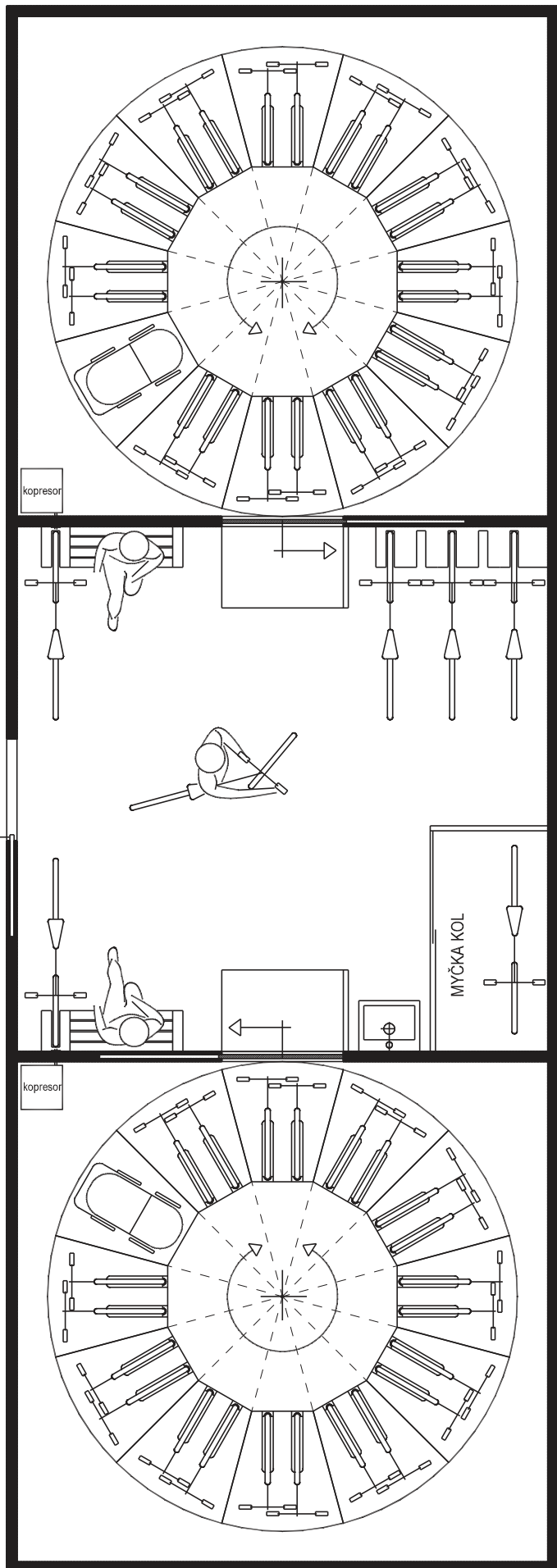
VARIANTA DISPOZIČNÍHO USPOŘÁDÁNÍ PRO BYTOVÉ DOMY
